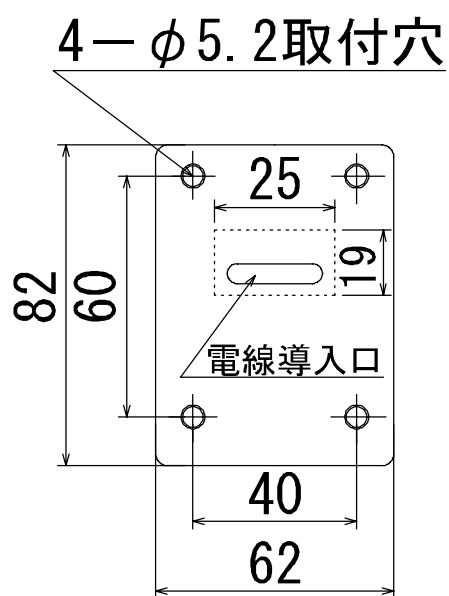
<<取付面 寸法図>>
